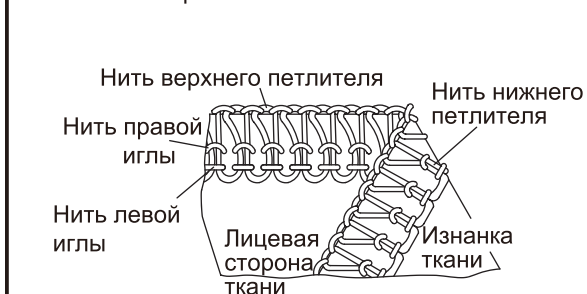
Нить правой иглы ослаблена и видна на изнаночной стороне ткани. Рис.5
