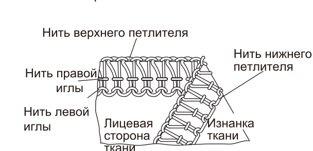
Нить левой иглы ослаблена и видна на изнаночной стороне ткани. Рис.4
