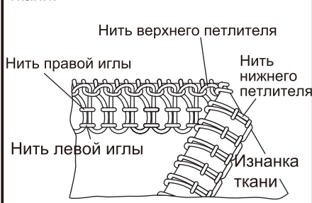
Нить нижнего петлителя перетянута на лицевую сторону ткани. Рис.3
