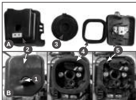
Рис. 14 Конструкция воздушного фильтра
