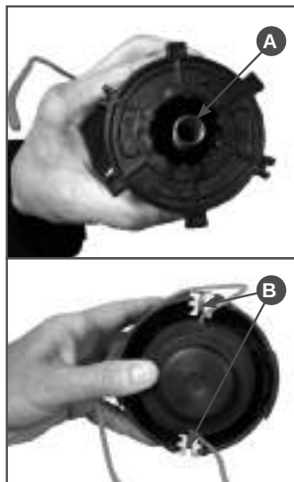
Рис. 18 Установка катушки в корпус
