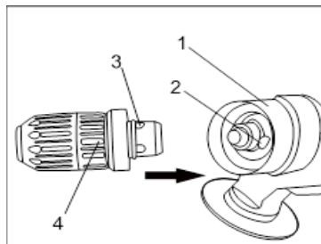
Рис.4. Установка быстрозажимного патрона
