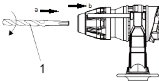
Рис. 3. Установка бура
