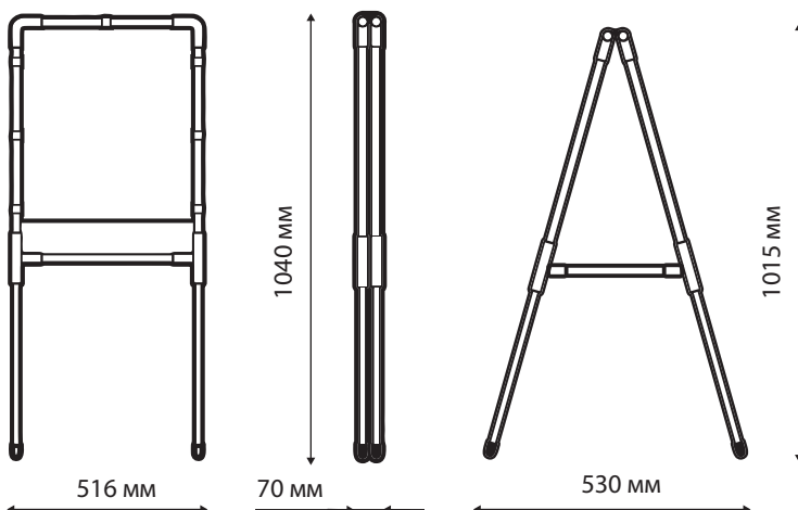
Рис. 2 Размеры мольберта, арт. М1
