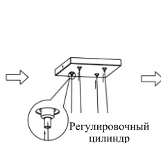
Прикрепите тросы к отверстиям потолочного кронштейна. Если Вы хотите отрегулировать высоту или вынуть установленные подвесные тросы, нужно опустить специальный регулирующий цилиндр вниз, а затем отрегулировать высоту или вынуть подвесные тросы.
