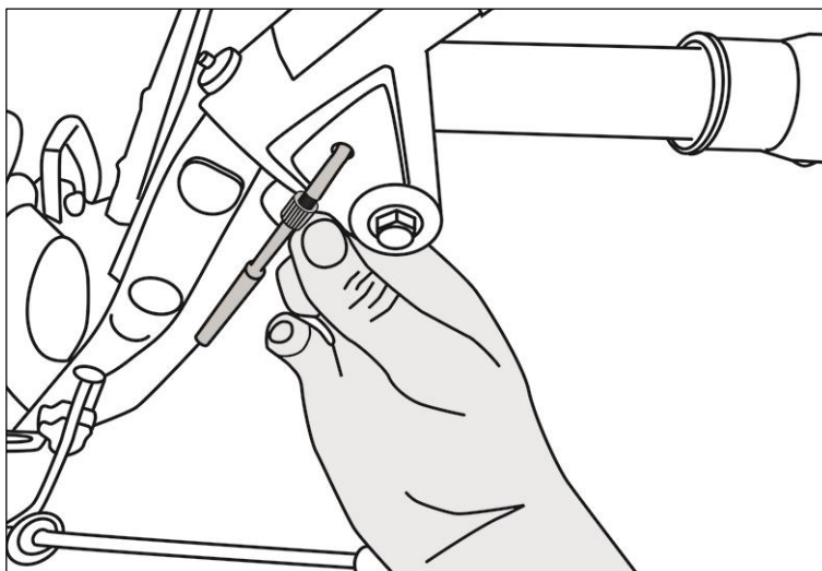
Рис. 8. Натяжка троса
