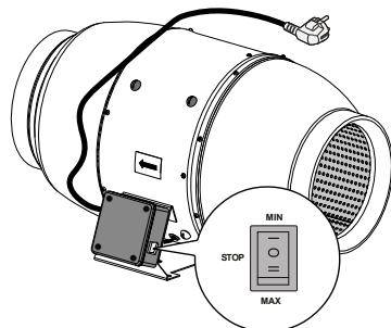
ТТ Сайлент-М ... П
