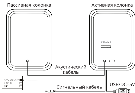
Рис. 2. Схема подключения
