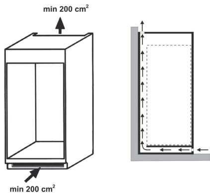
Рисунок Б.5 - Схема циркуляции воздуха вокруг холодильного прибора Сурет Б.5 - Тоңазытқыш прибор айналасындағы ауа айналысының схемасы
