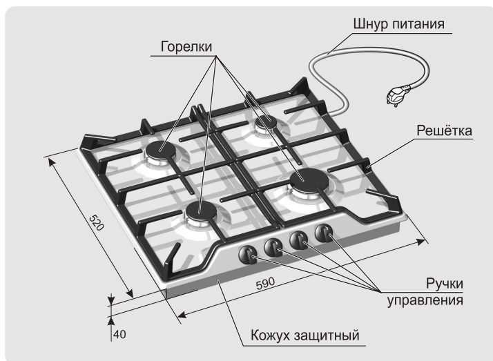
Рис. 1 МОДЕЛЬ ПВГ 1212
