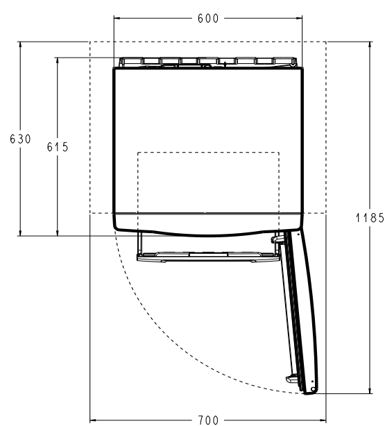
Андозаи кори асбоби хунуккунанда.
