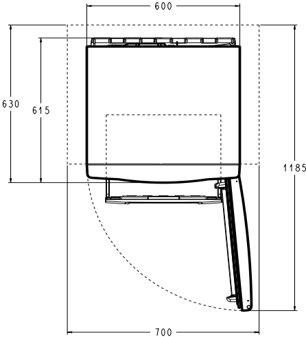
Хөргөх төхөөрөмжийн ажлын хэмжээ
