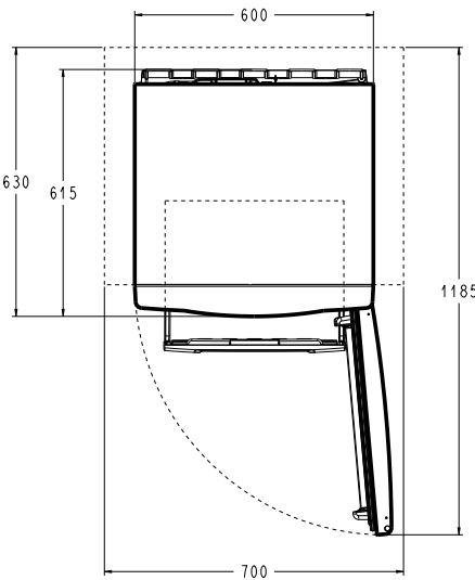
Sovutish qurilmasining ishchi oʻlchamlari.
