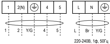
Внутренний блок модели ASW-H24B4/FJ-R1
