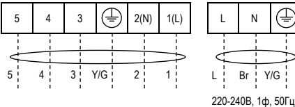
Внутренний блок модели ASW-H24B4/FJ-R1
