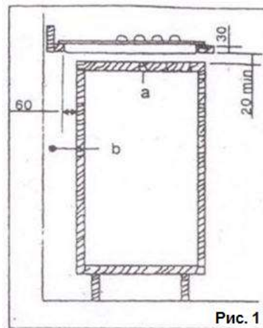
a съемная стенка b пространство для подключения
