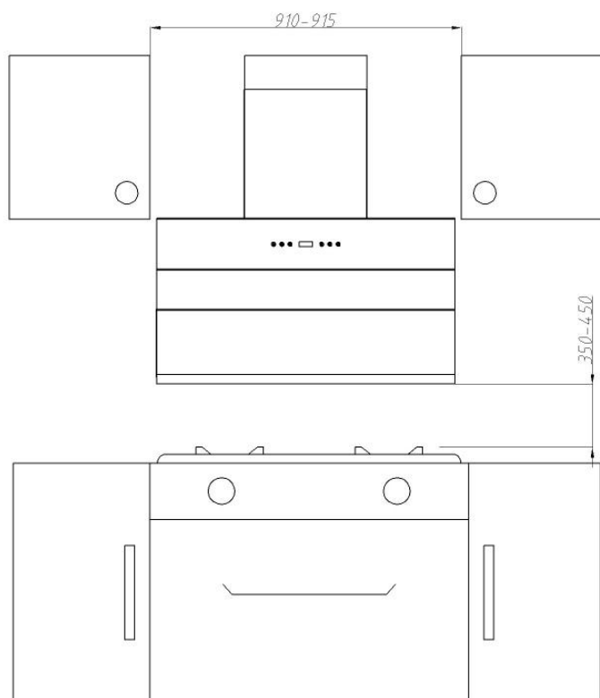
Рисунок 1-А. Отдельностоящий прибор
