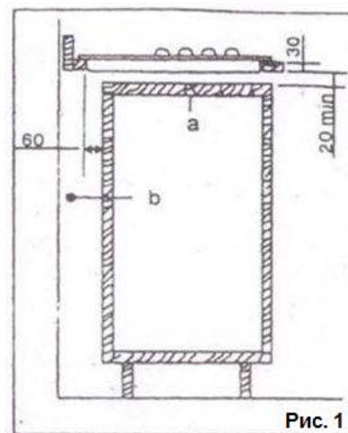
a съемная стенка b пространство для подключения
