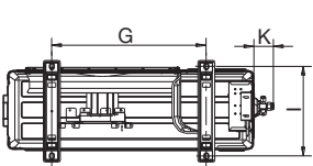
Наружный блок
