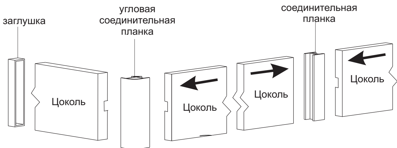
Соединение цоколя планками
