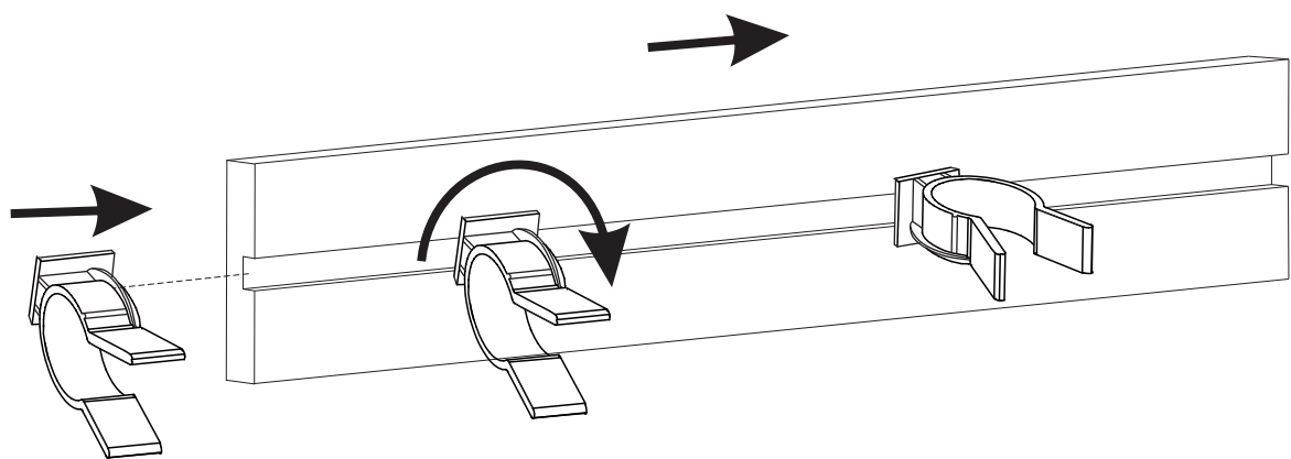
Соединение клипс с цоколем
