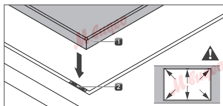
рис. 10.14 Установка пластин для выравнивания по высоте
