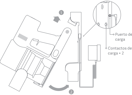
Cargar la aspiradora en el soporte de carga
