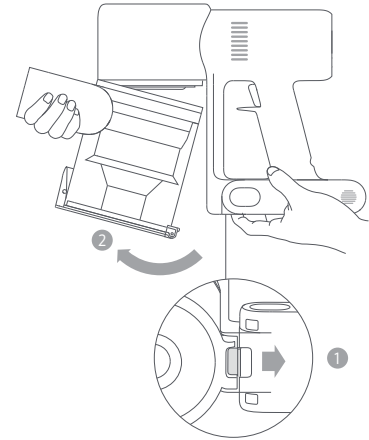
Bouton de déverrouillage du compartiment à poussière
