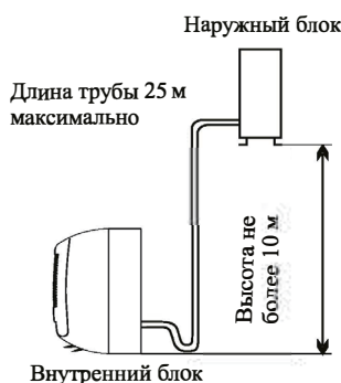
Схема установки
