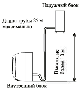
Схема установки
