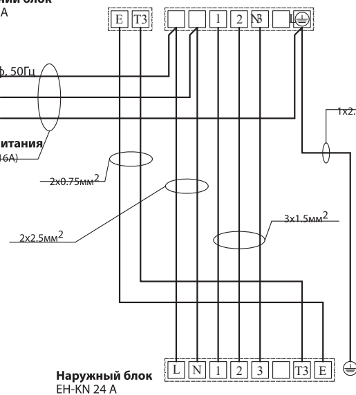
Внутренний блок EH-KN 24 A
