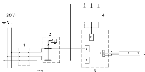
Рисунок 5: Электросхема
