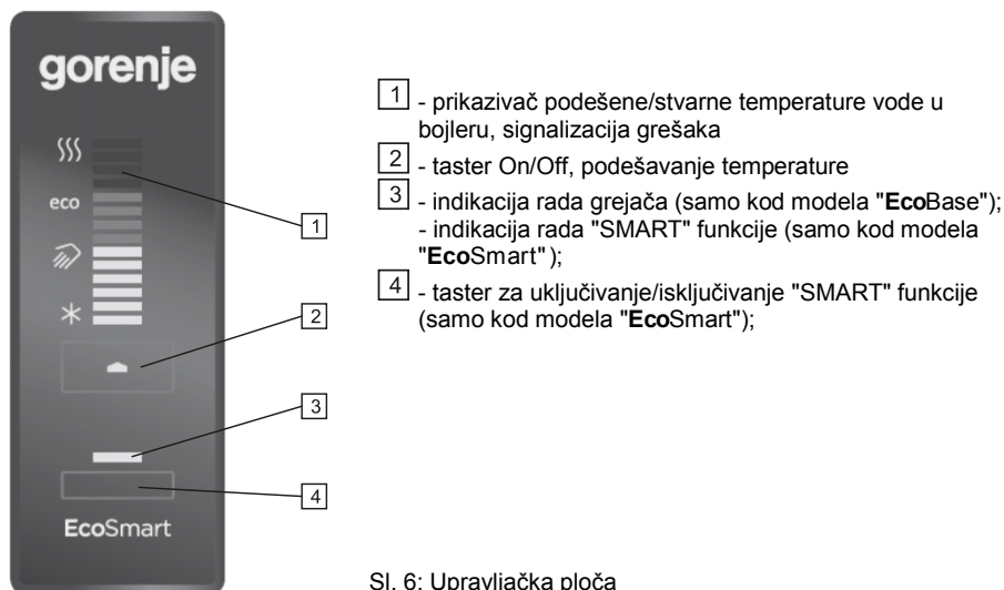
Sl. 6: Upravljačka ploča
