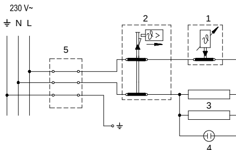
Instalația electrică
