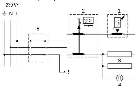
Электросхема
