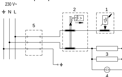
Электросхема
