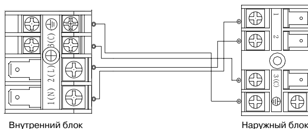
Внутренний блок
