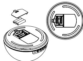
Установка аккумуляторных батарей
