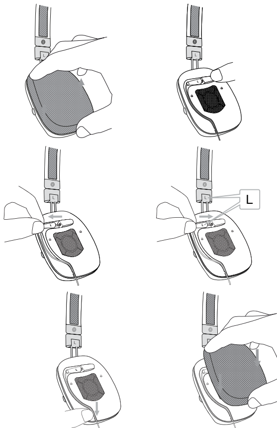
4. Ábra A vezeték cseréje
