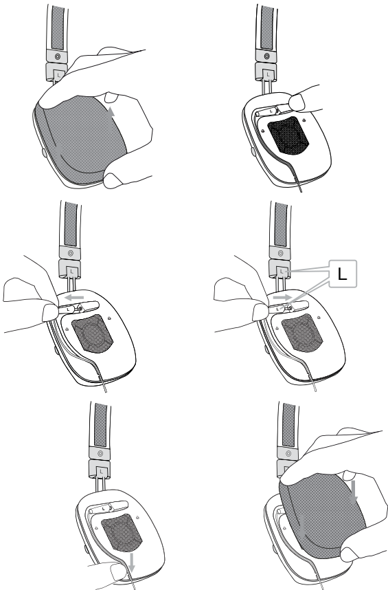
图4 更换接线
