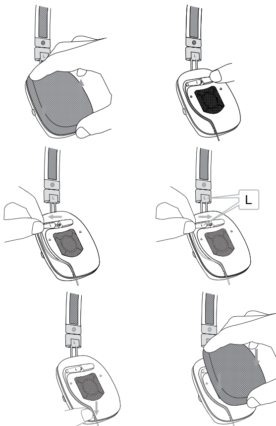
Diagrama 4 Substituindo o cabo
