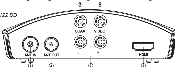
Рис. 3. Задние панели EASY SEE-121 и EASY SEE-122 DD
