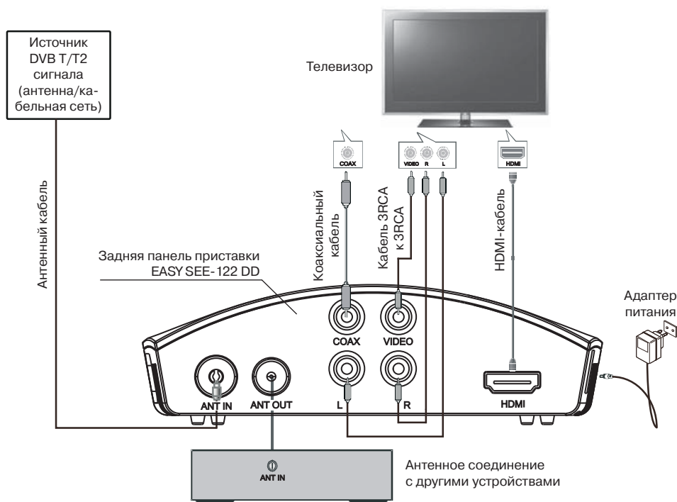
Рис. 5. Схема подключения
