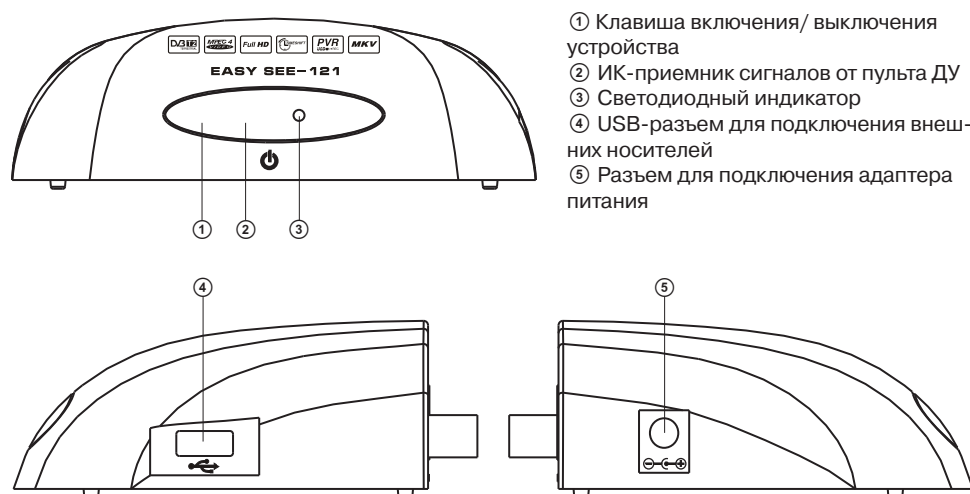
Рис. 1. Лицевая и боковые панели EASY SEE-121
