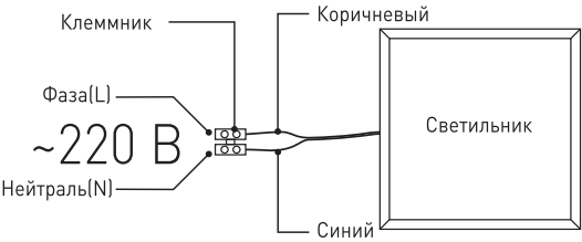
Рис.1. Схема подключения светильника к сети 220В.
