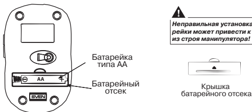
Рис. 4. Установка батареек
