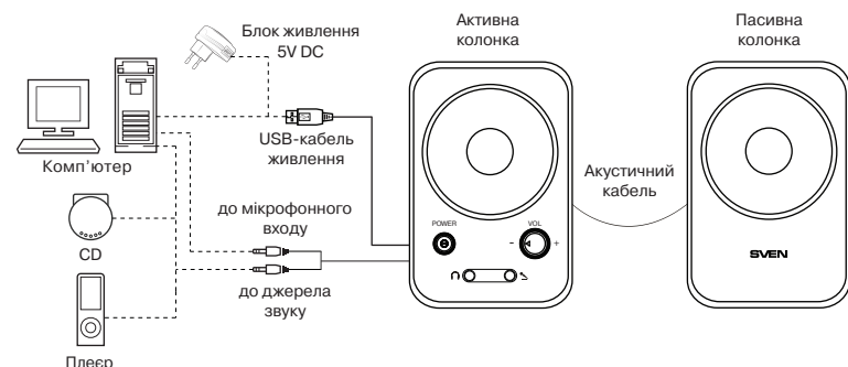
Мал. 2. Схема підключення
