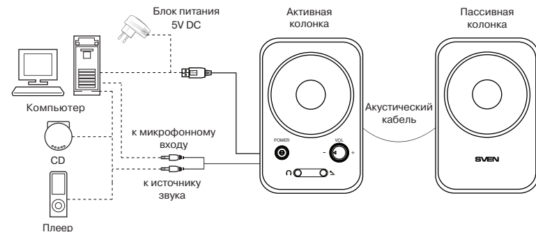
Рис. 2. Схема подключения
