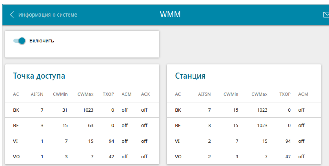
Рисунок 102. Страница для настройки функции WMM.
