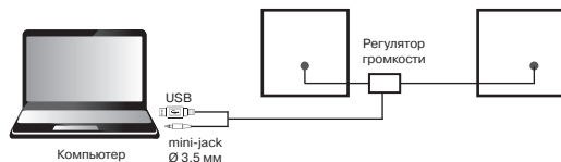
Схема подключения
