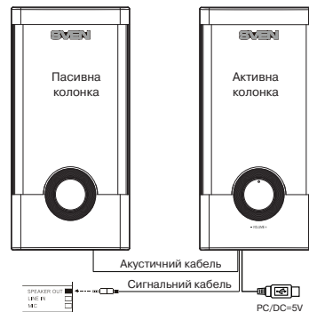
Мал. 2. Схема підключення
