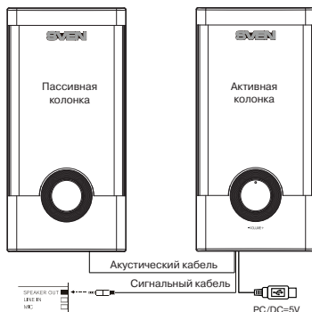
Рис. 2. Схема подключения
