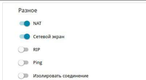
Рисунок 68. Страница добавления соединения типа PPPoE . Раздел Разное .
