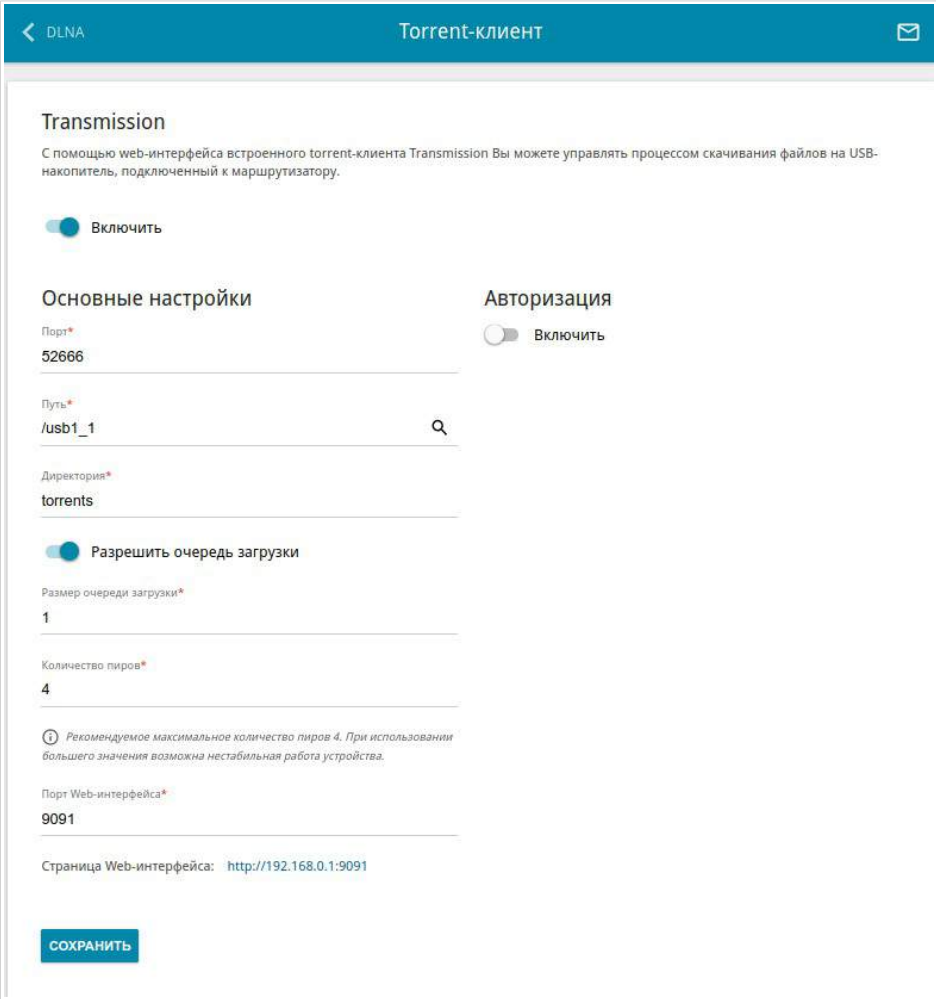
Рисунок 119. Страница USB-накопитель / Torrent-клиент .
