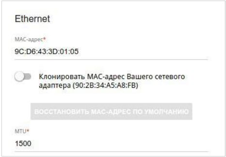
Рисунок 57. Страница добавления соединения типа Статический IPv4 . Раздел Ethernet .
