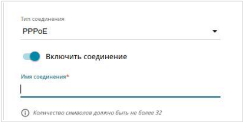
Рисунок 65. Страница добавления соединения типа PPPoE. Выбор типа соединения.
