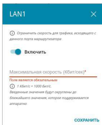
Рисунок 137. Окно для настройки ограничения скорости.
