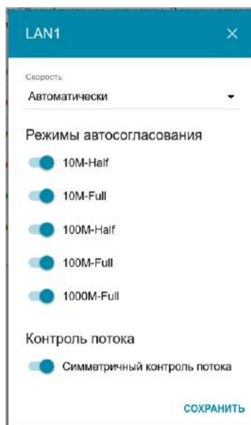
Рисунок 135. Окно изменения настроек порта маршрутизатора.
