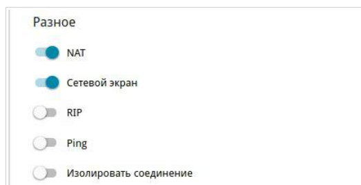
Рисунок 60. Страница добавления соединения типа Статический IPv4 . Раздел Разное .
