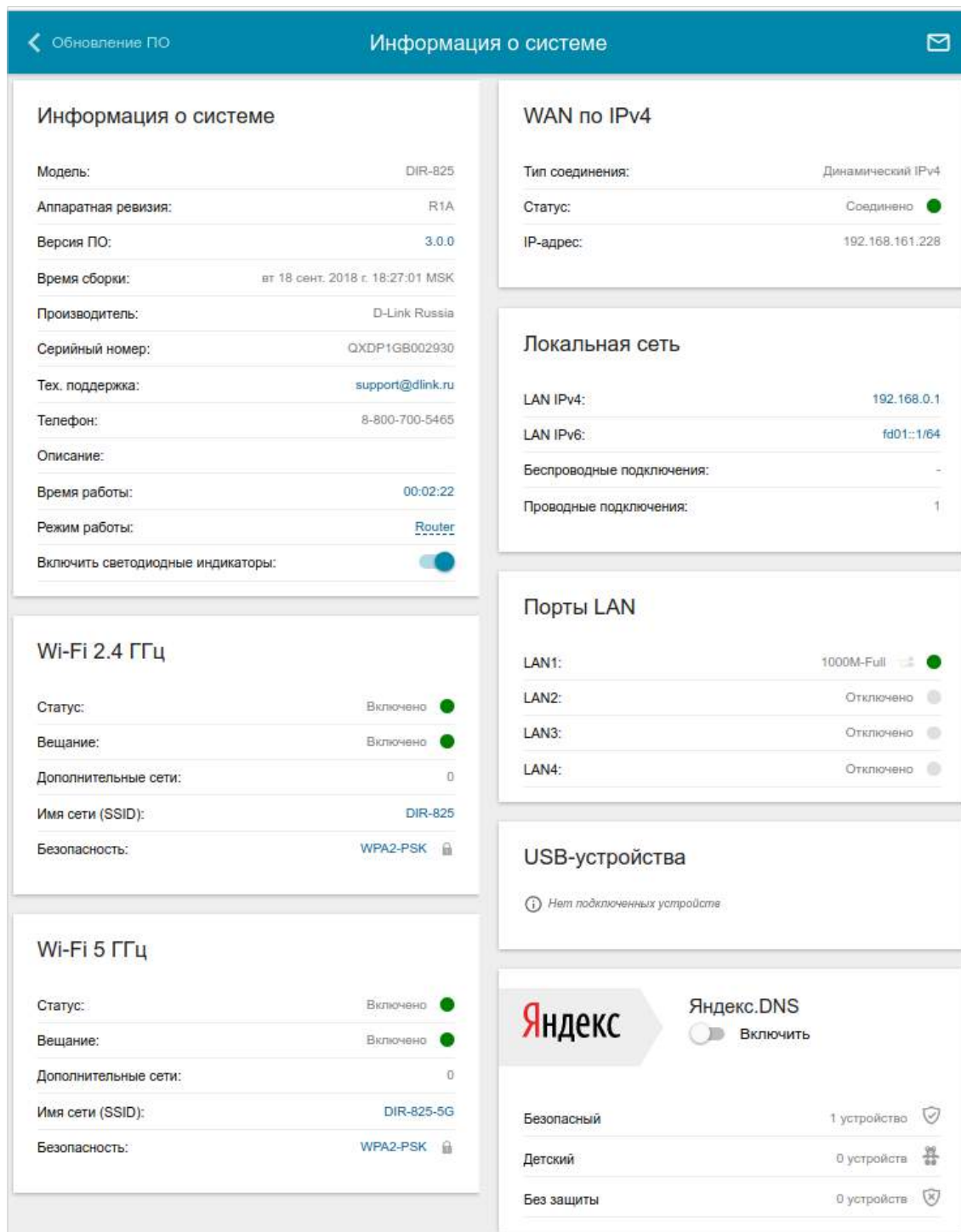
Рисунок 15. Страница информации о системе.
