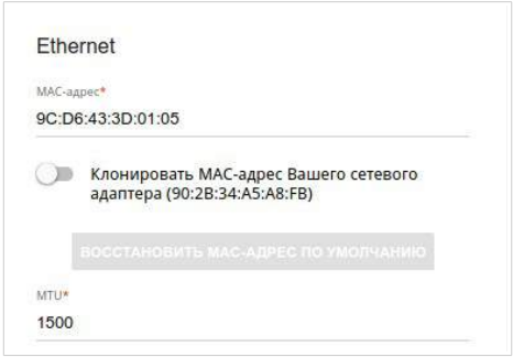
Рисунок 62. Страница добавления соединения типа Статический IPv6 . Раздел Ethernet .
