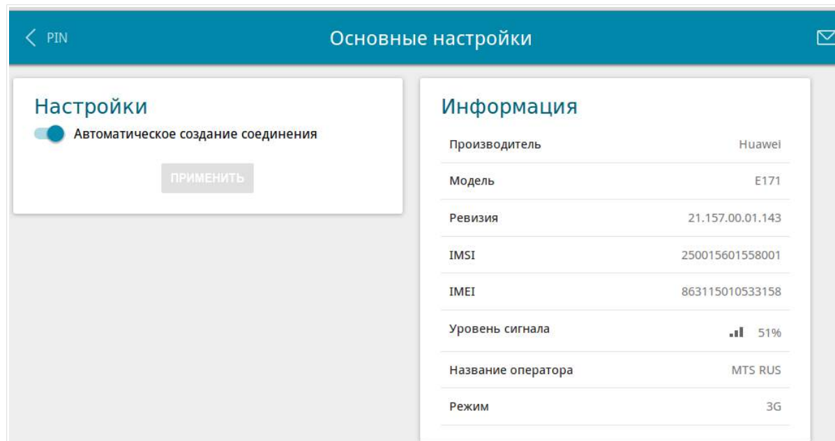
Рисунок 125. Страница USB-модем / Основные настройки .
