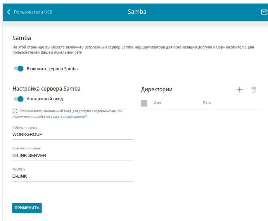
Рисунок 113. Страница USB-накопитель / Samba .
