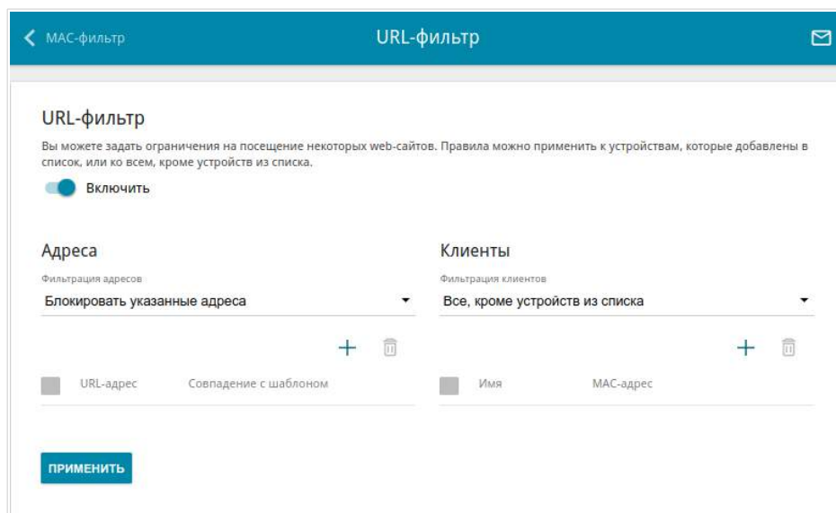
Рисунок 161. Страница Межсетевой экран / URL-фильтр .
