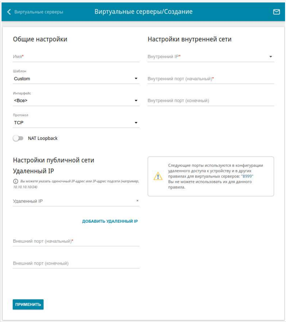
Рисунок 157. Страница добавления виртуального сервера.
