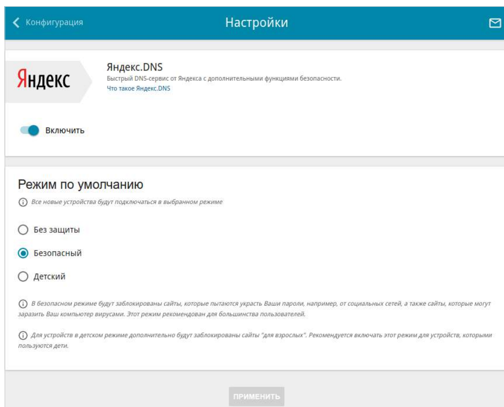
Рисунок 173. Страница Яндекс.DNS / Настройки .
