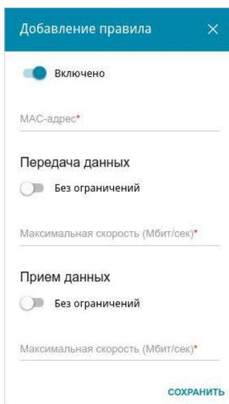
Рисунок 104. Окно для настройки ограничения скорости.
