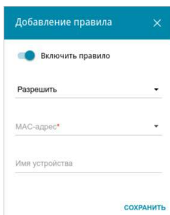
Рисунок 160. Окно добавления правила для MAC-фильтра.
