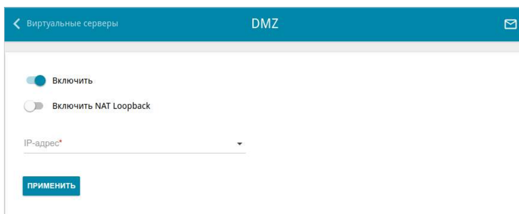
Рисунок 125. Страница Межсетевой экран / DMZ .
