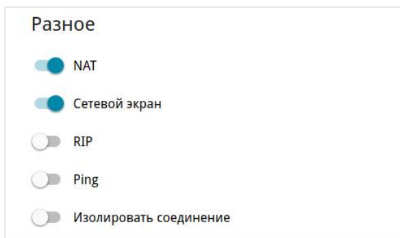
Рисунок 59. Страница добавления соединения типа Статический IPv4 . Раздел Разное .
