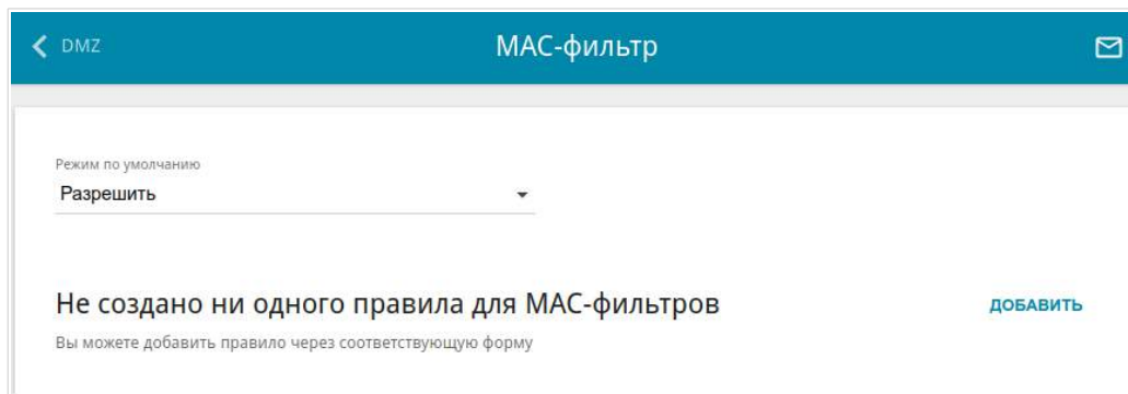
Рисунок 126. Страница Межсетевой экран / MAC-фильтр .
