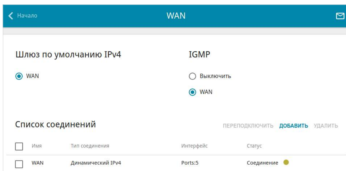
Рисунок 54. Страница Настройка соединений / WAN .
