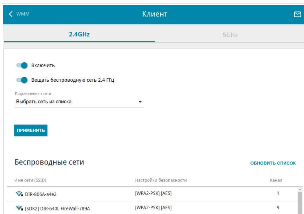
Рисунок 92. Страница для настройки маршрутизатора в качестве клиента.
