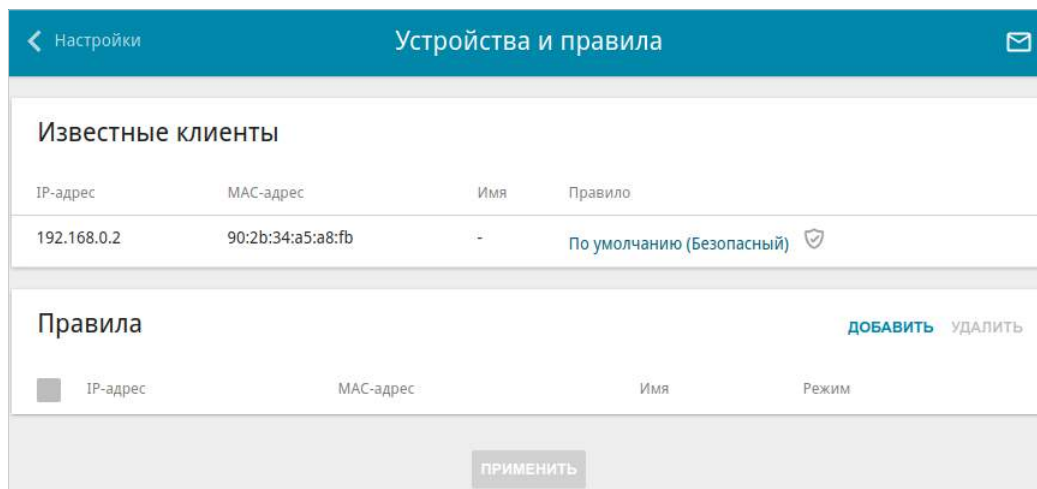
Рисунок 140. Страница Яндекс.DNS / Устройства и правила .
