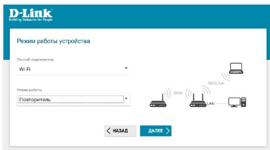
Рисунок 28. Выбор режима работы устройства. Режим Повторитель .
