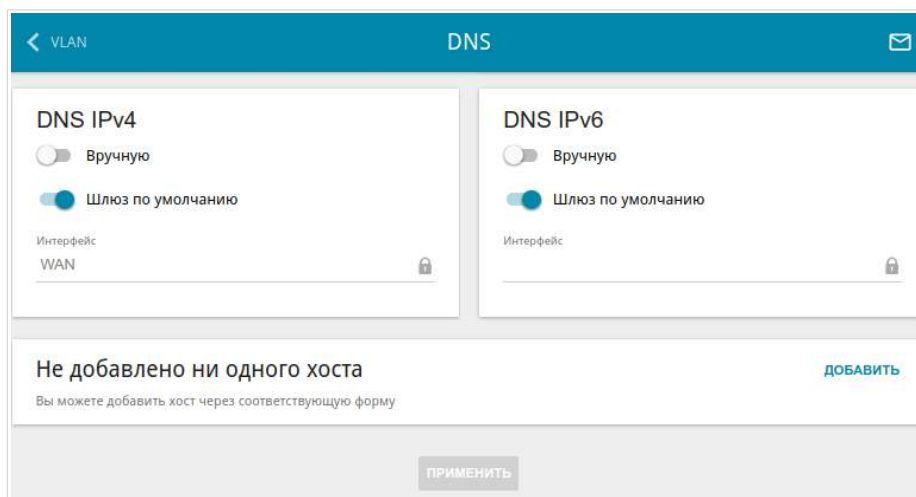
Рисунок 99. Страница Дополнительно / DNS .
