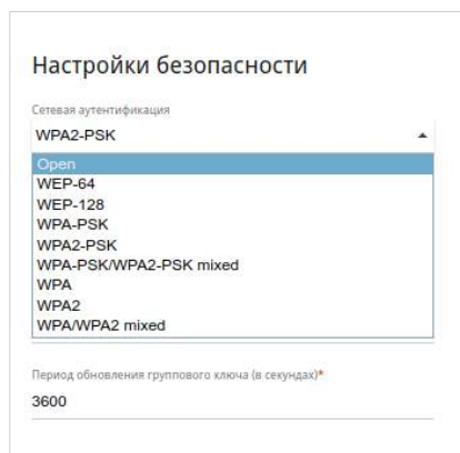
Рисунок 84. Типы аутентификации, поддерживаемые маршрутизатором.
