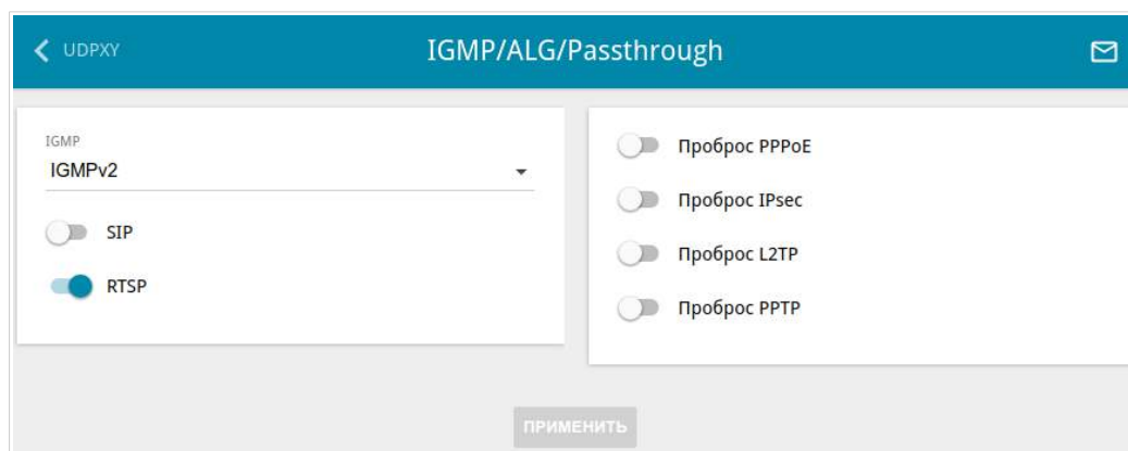
Рисунок 116. Страница Дополнительно / IGMP/ALG/Passthrough .
