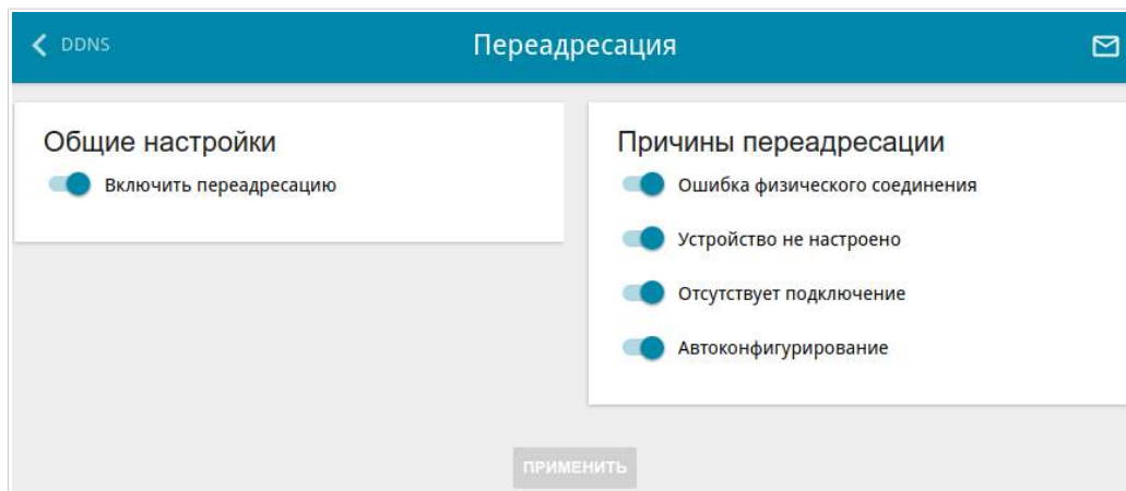
Рисунок 107. Страница Дополнительно / Переадресация .
