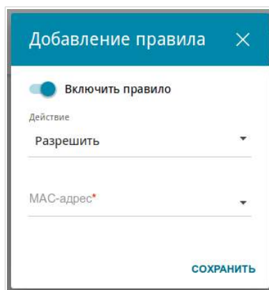
Рисунок 127. Окно добавления правила для MAC-фильтра.
