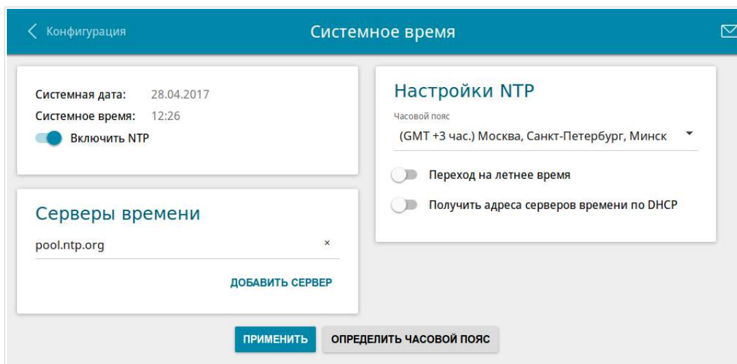
Рисунок 138. Страница Система / Системное время .
