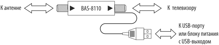
Рисунок 1. Типовая схема подключения усилителя
