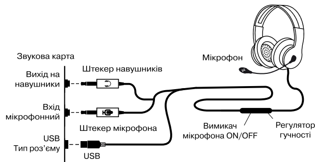
Мал. 1. Схема підключення
