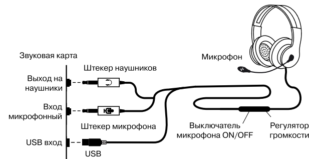
Рис. 1. Схема подключения
