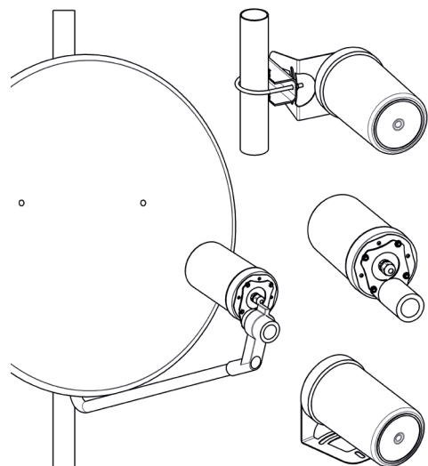
РИСУНОК 3. ВАРИАНТЫ УСТАНОВКИ ВНЕШНЕГО БЛОКА
