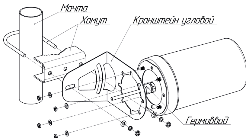
РИСУНОК 2. МОНТАЖ ВНЕШНЕГО БЛОКА НА МАЧТУ
