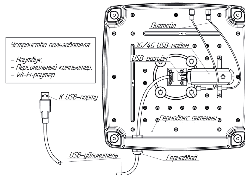
РИСУНОК 4. СХЕМА ПОДКЛЮЧЕНИЯ УСТРОЙСТВА
