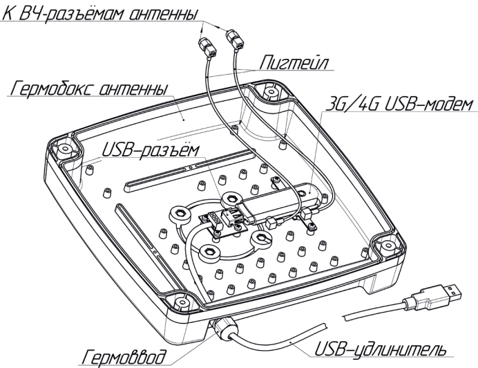
РИСУНОК 1. УСТАНОВКА И ПОДКЛЮЧЕНИЕ USB-МОДЕМА
