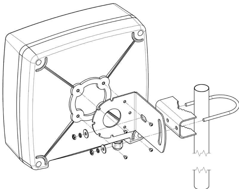
РИСУНОК 2. МОНТАЖ ВНЕШНЕГО БЛОКА НА МАЧТУ
