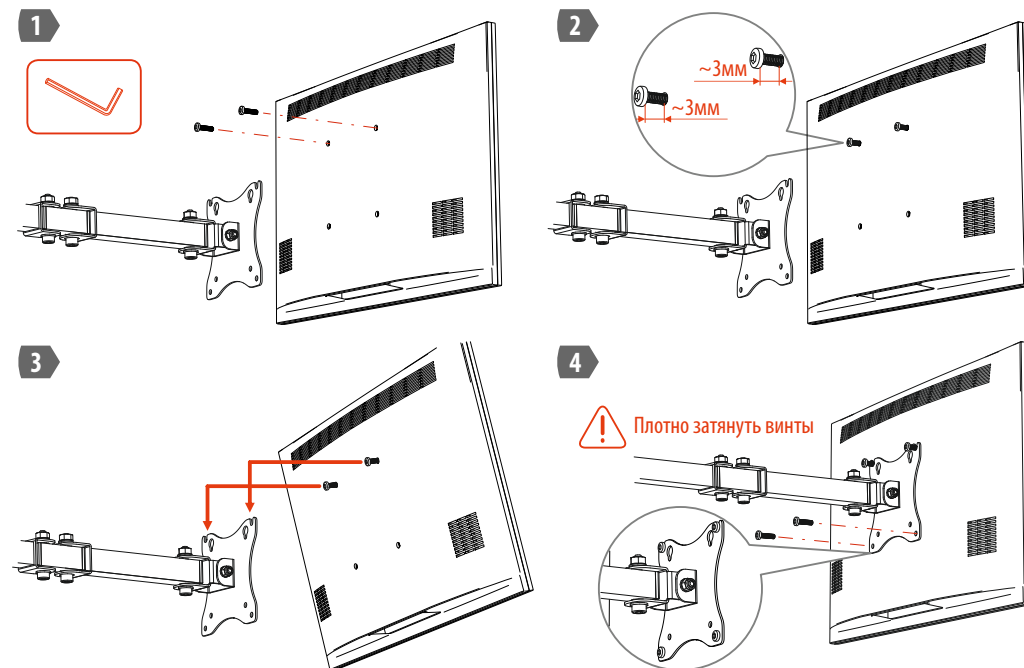
Рисунок 2. Монтаж телевизора/монитора на держатель
