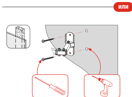
Рисунок 1. Установка кронштейна на стену
